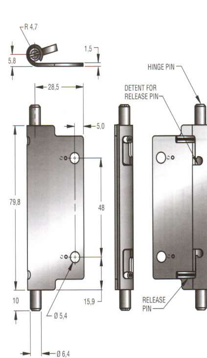
Door Leaf
