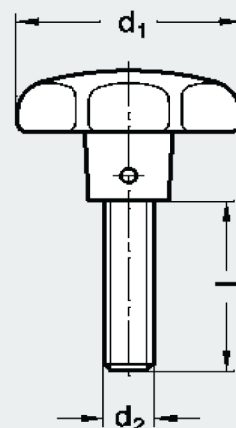
• Type SG Hand knob DIN 6336 Type E Cast iron (GG)
