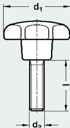
Type ST Hand knob DIN 6336 Type K Plastic (KT) Technopolymer (PA)
