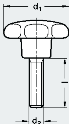
Type SK Hand knob DIN 6336 Type K Plastic (KU) Duroplast (PF)
